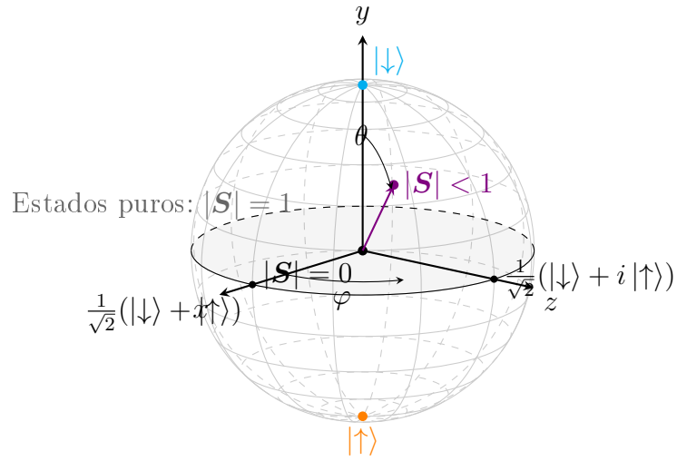
Figura A.1: Esfera de Bloch para un sistema de espín 1/2 . Los estados puros corresponden a la superficie ( |\mathbf{S}| = 1 ), los estados mixtos al interior ( |\mathbf{S}| < 1 ) y el estado completamente mezclado al origen ( |\mathbf{S}| = 0 ).
